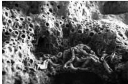
汐吹崎南 隆起貝層
