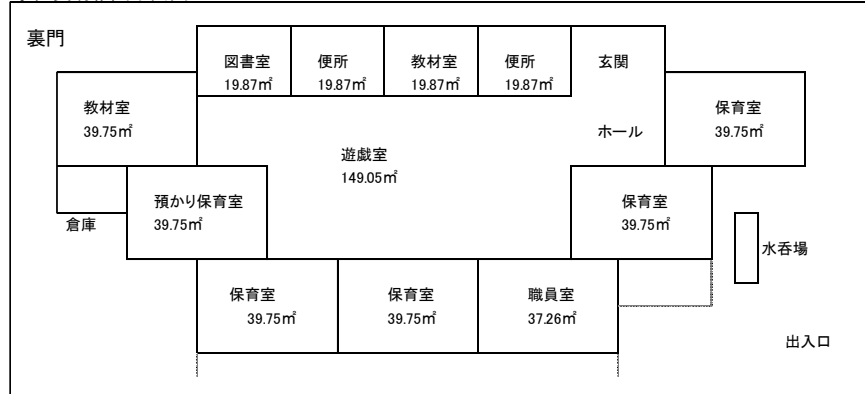
宇佐美幼稚園平面図
