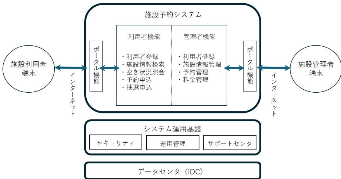
「図 1-7 システムの全体概要」
